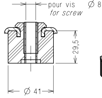
Detail suspension Echelle : 1/2 Scale : 1/2
