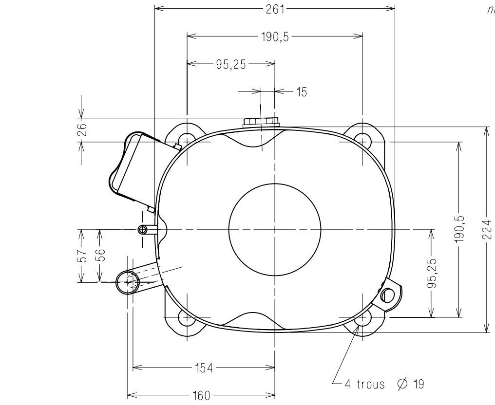
Detail suspension Echelle : 1/2 Scale : 1/2
