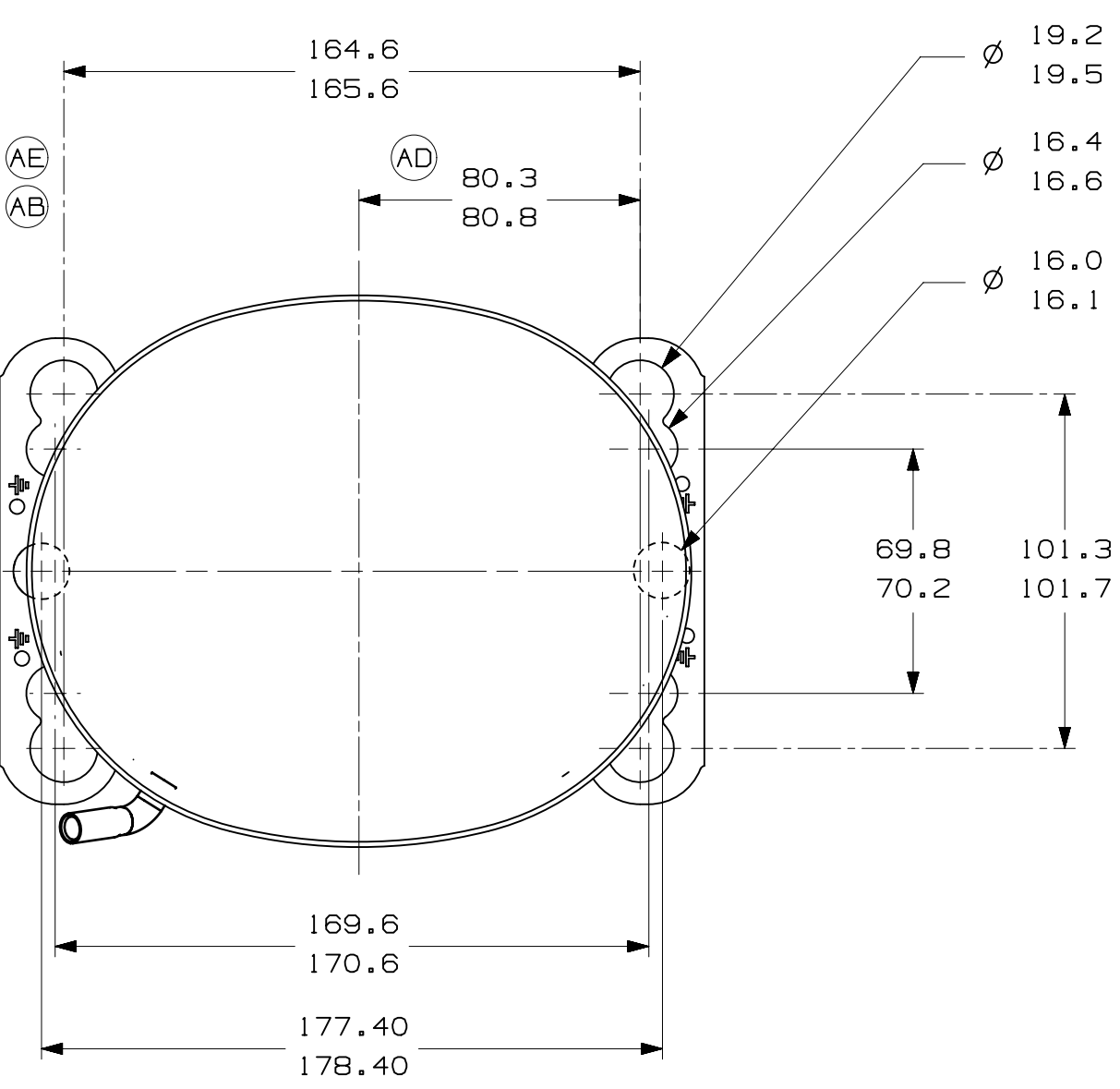
-VISTA AUXILIAR- DIMENSOES DE FIXACAO
