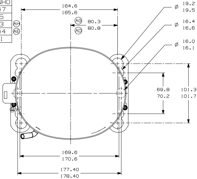
-VISTA AUXILIAR- DIMENSOES DE FIXACAO
