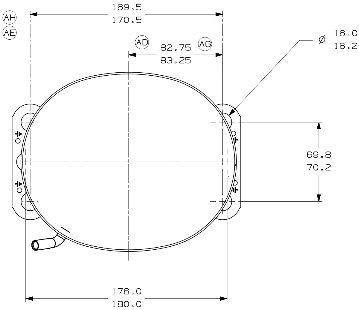
-VISTA AUXILIAR- DIMENSOES DE FIXACAO
