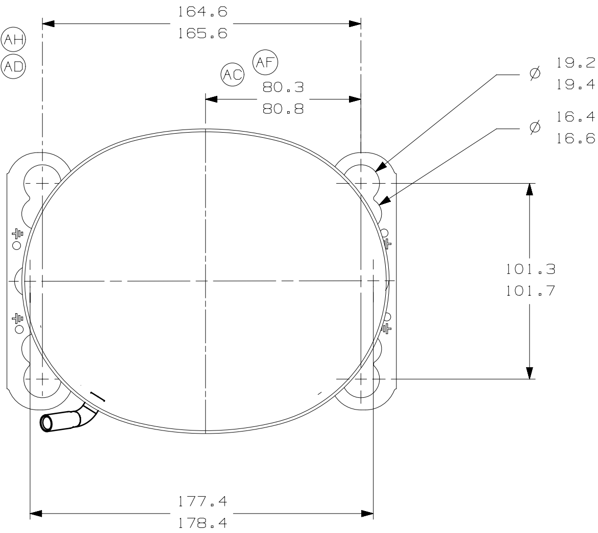
-VISTA AUXILIAR- DIMENSOES DE FIXACAO
