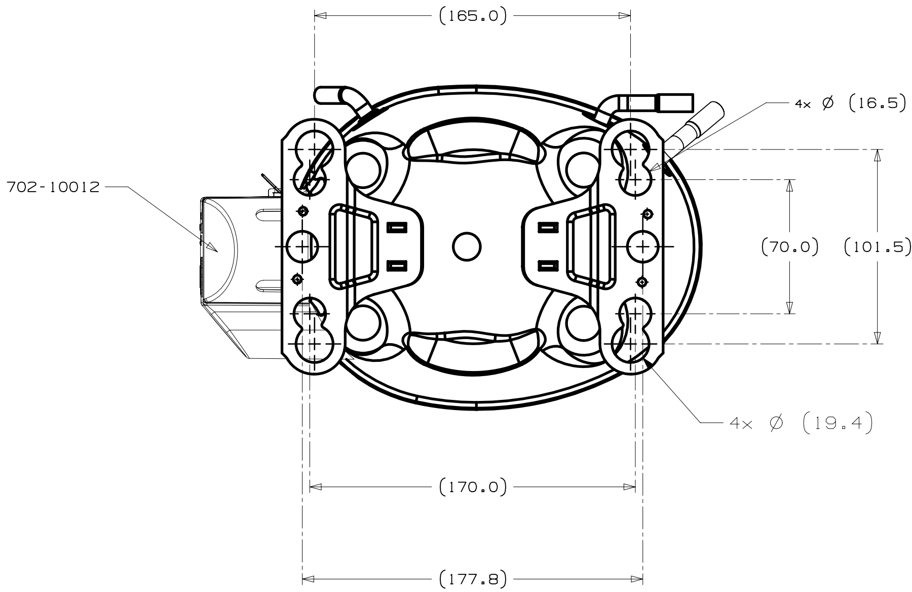
VISTA AUXILIAR DIMENSOES DE FIXACAO
