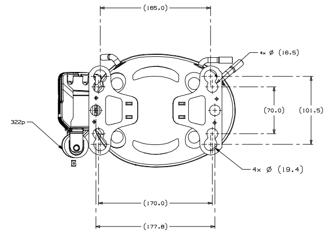
VISTA AUXILIAR DIMENSÕES DE FIXAÇÃO
