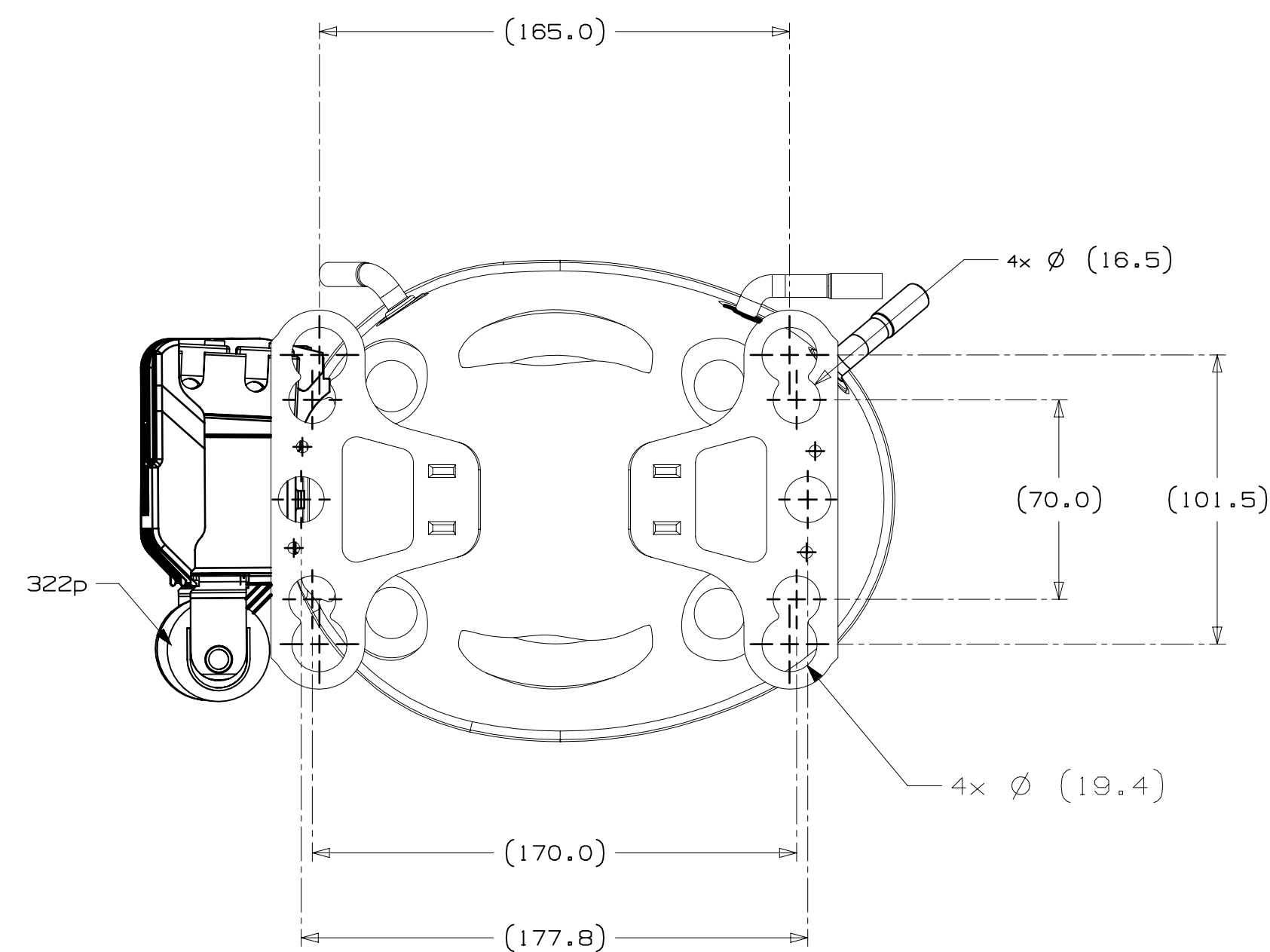
VISTA AUXILIAR DIMENSOES DE FIXACAO
