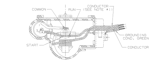
T. I. RELAY SHOWN NO FAN
