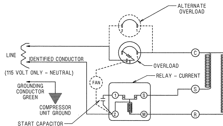
115 OR 230 VOLT - SCHEMATIC WIRING DIAGRAM - CSIR REF. DWG. MD472-1
