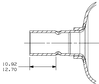
(AD) CORTE A-A ESCALA 2:1
