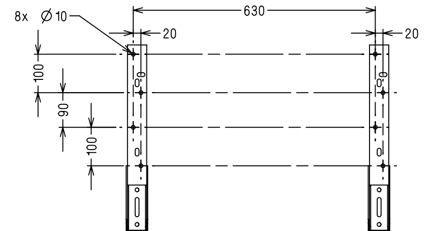
MONTAGE AU MUR WALL MOUNTING
