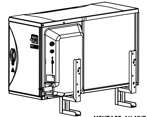
MONTAGE AU MUR WALL MOUNTING
