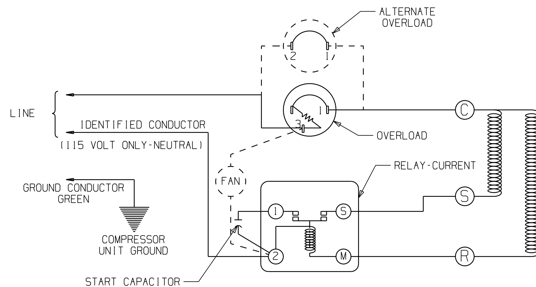
115 OR 230 VOLT -SCHEMATIC WIRING DIAGRAM-CSIR REF. DWG. MD-472-1
