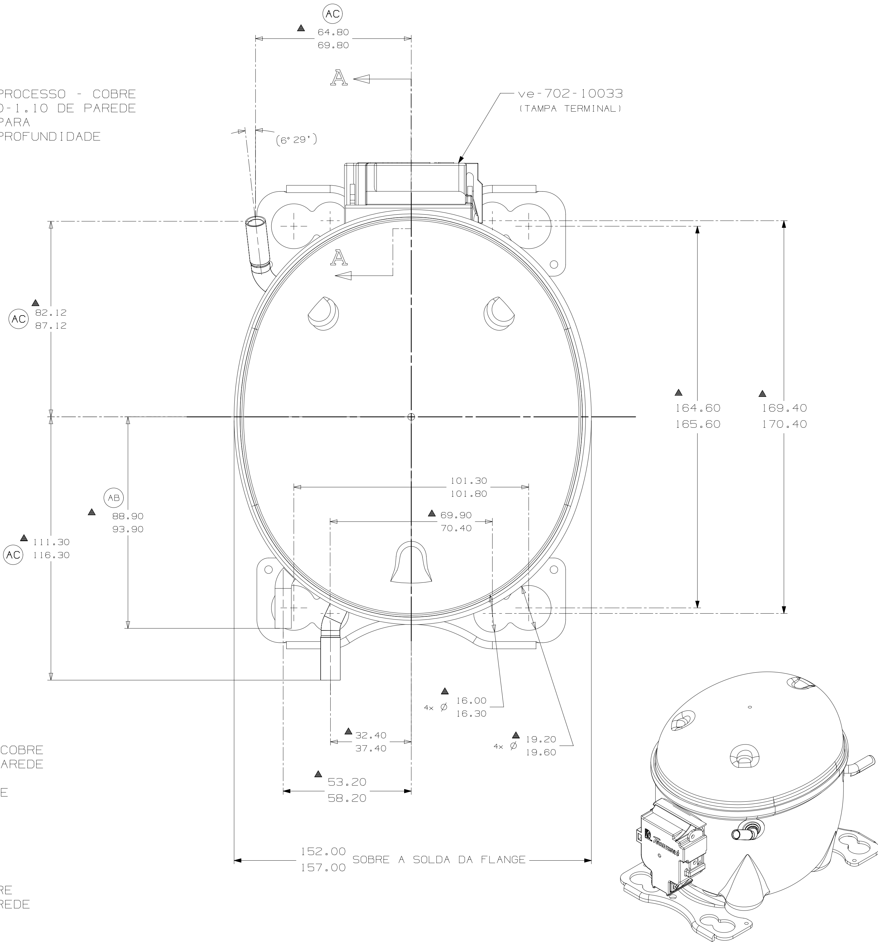
VISTA PERSPECTIVA ESCALA 1:2
